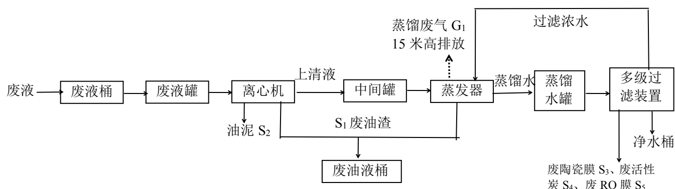
图 3.6-1 工艺流程图
